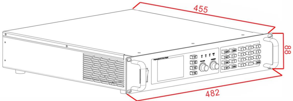
图 1-3 外形尺寸图
