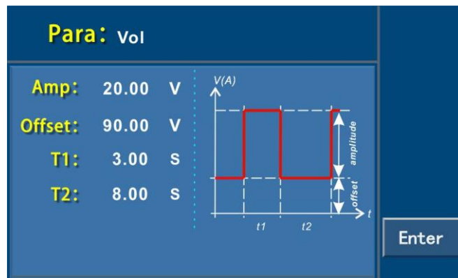
图 3-31 输出矩形波
