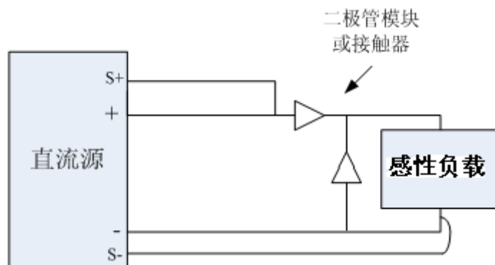
图 2-3 感性负载接线方式
