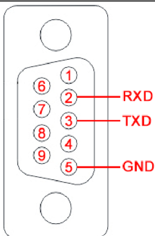
RS232 接口定义
