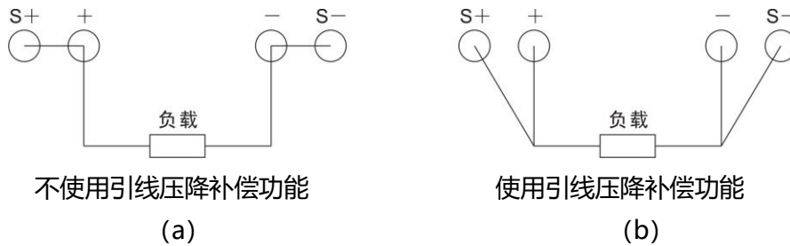
图 2-1 输出接线示意图
