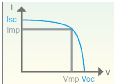
图 3-33 I-V 模式输出曲线
