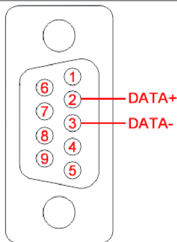
RS485 接口定义
