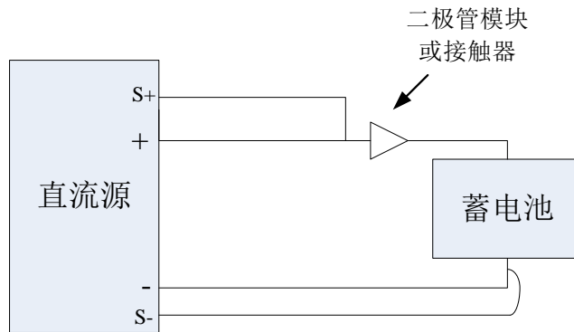
图 2-2 蓄电池负载接线方式
