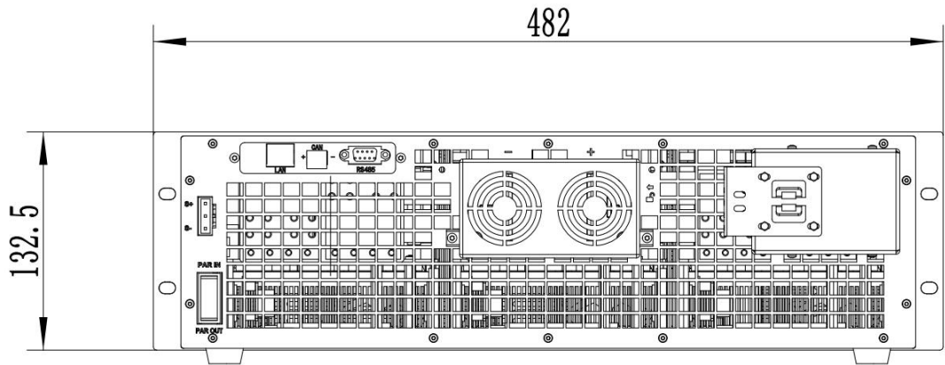
图 1-9 后视图
