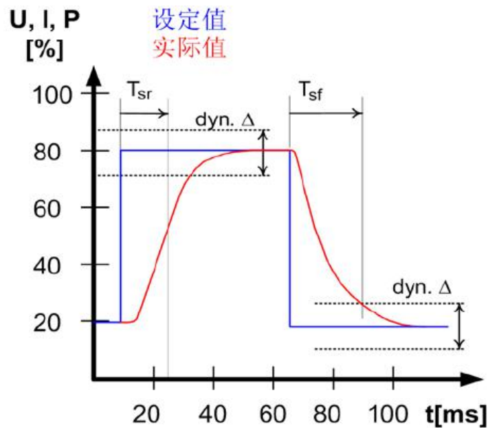
图 3-7-5 阶跃响应报警曲线示意图
