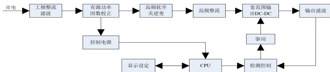
图 1-1 原理示意图
