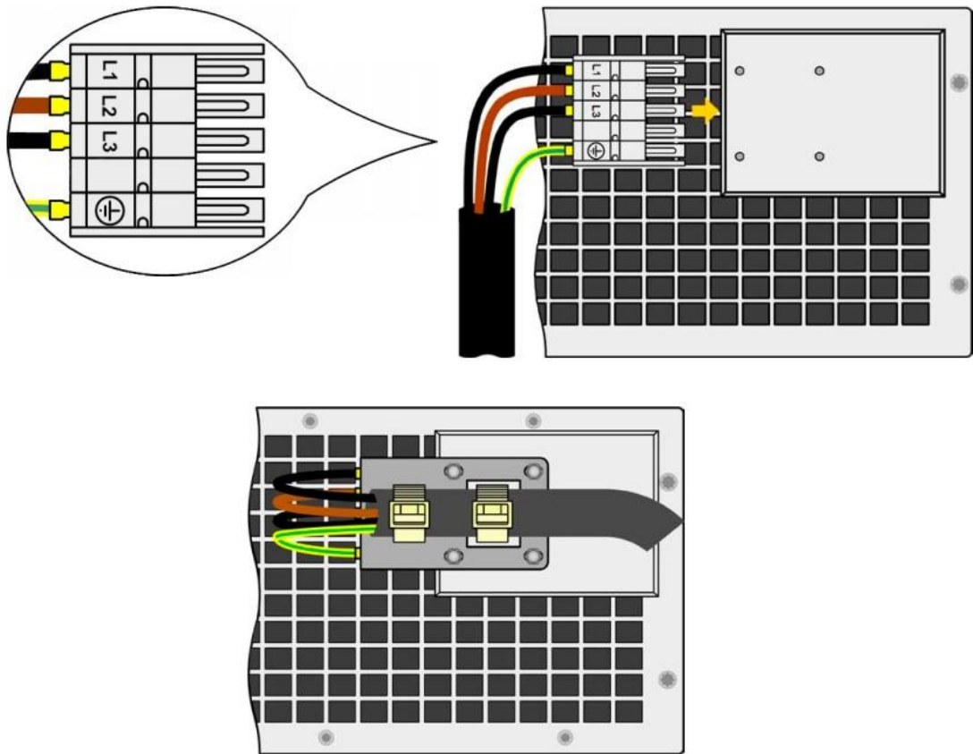
图 2-1 后面板输入接线端子示意图
