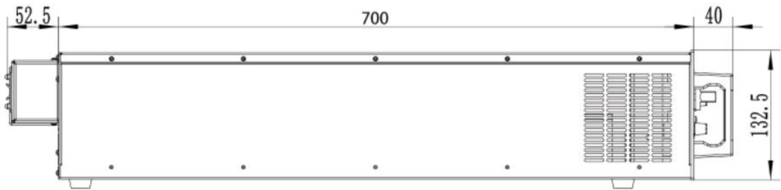
图 1-10 右视图
