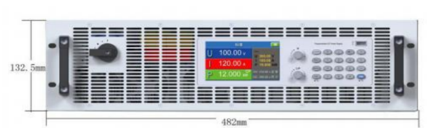
图 1-8 正视图
