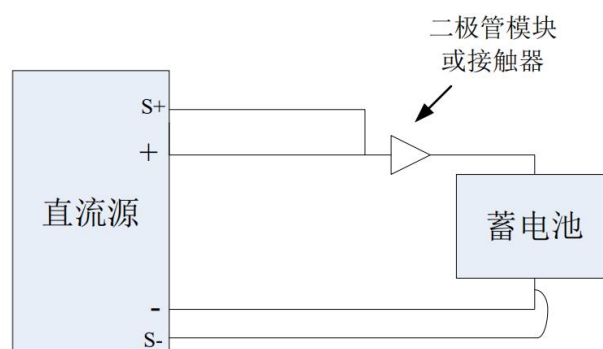
图 2-4 蓄电池负载接线方式
