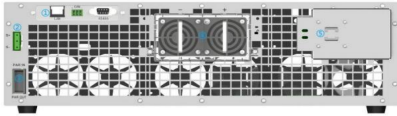
图 1-13 后面板示意图
