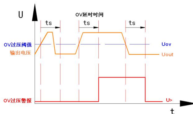
图 1-5 OV 过压警报工作示意
