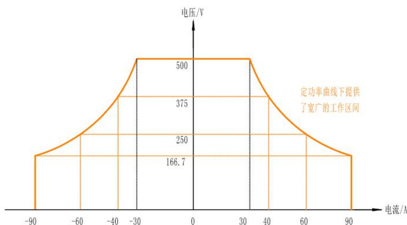
图 1-2 PSB系列双向可编程电源输出特性曲线
